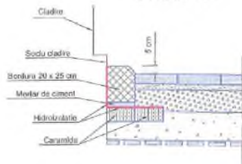
Detaliul "A"
