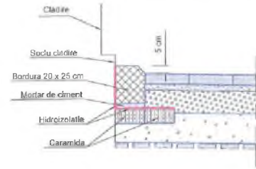
Detaliul "A"
